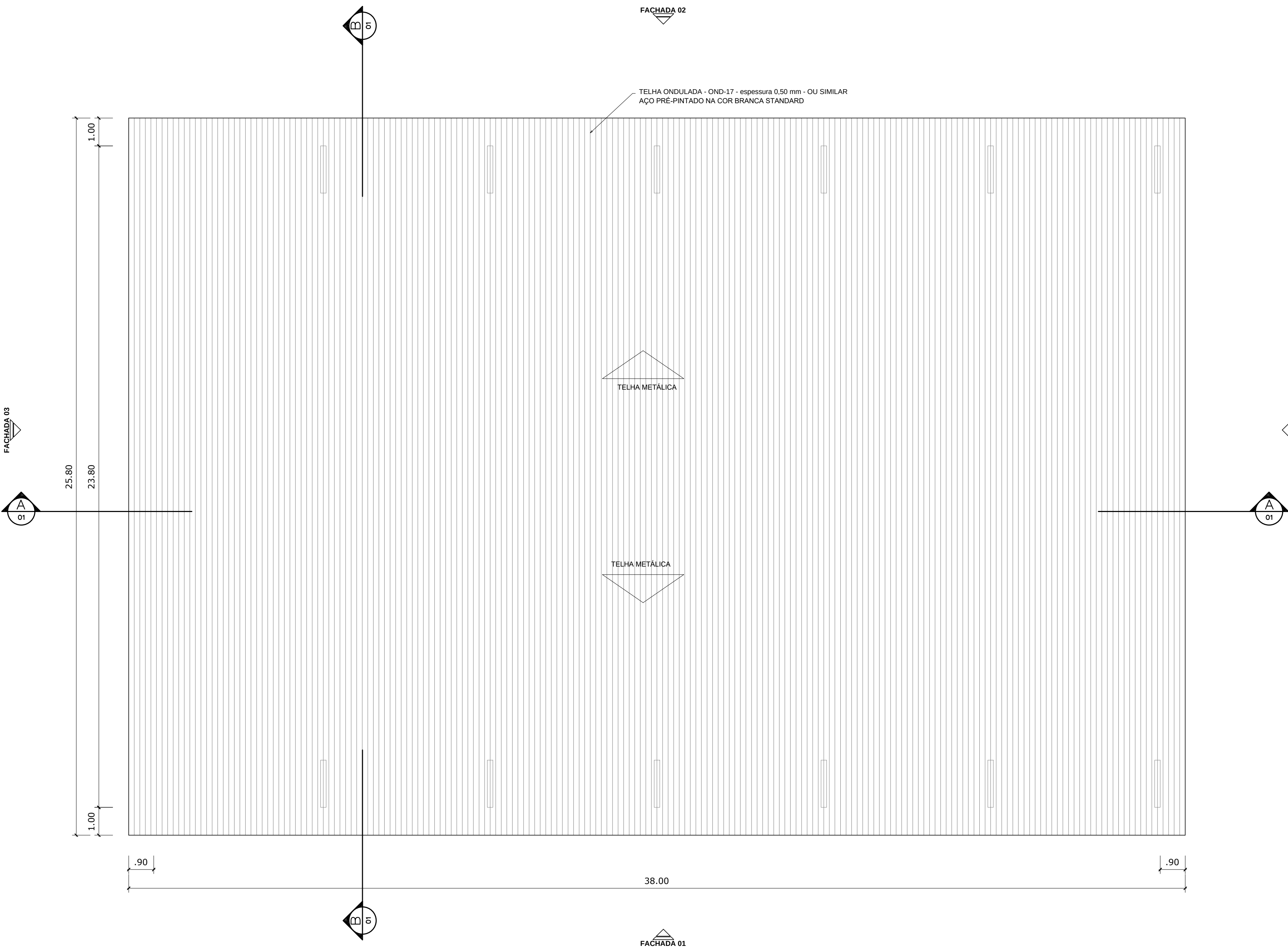
PLANTA DE COBERTURA ESCALA 1:125
