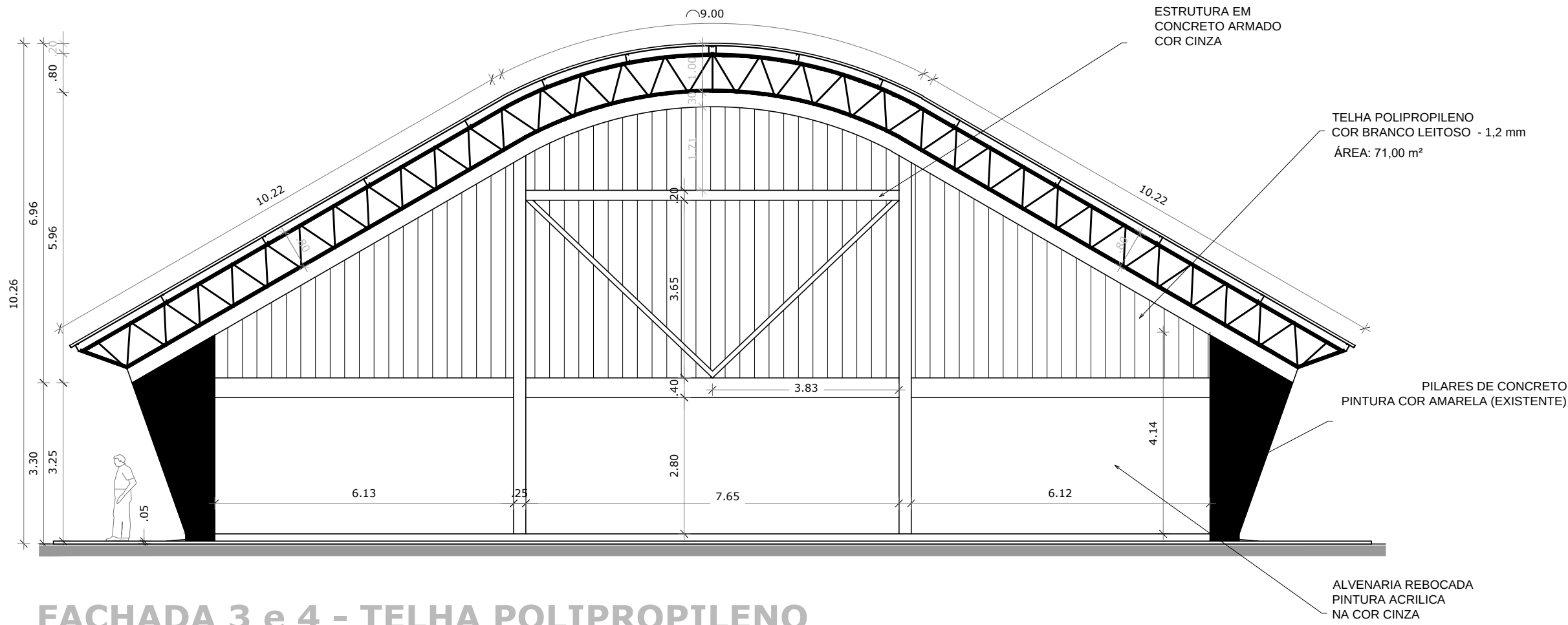
FACHADA 3 e 4 - TELHA POLIPROPILENO ESCALA 1:150
