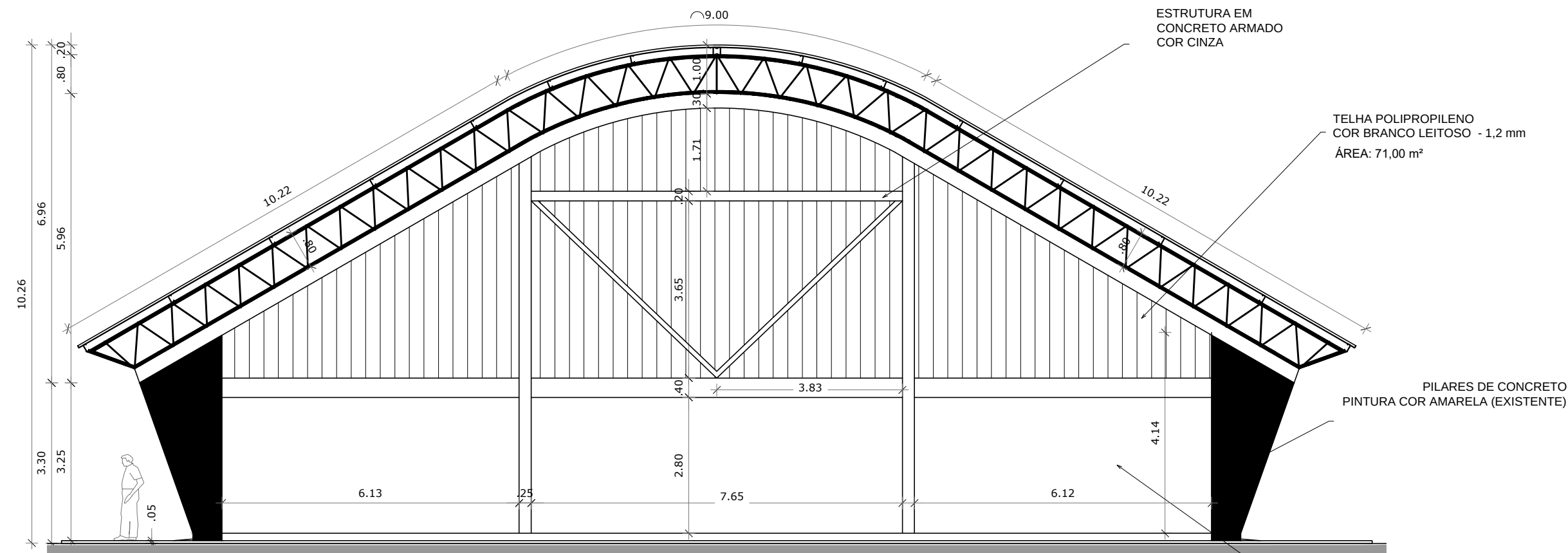
FACHADA 3 e 4 - TELHA POLIPROPILENO ESCALA 1:150
