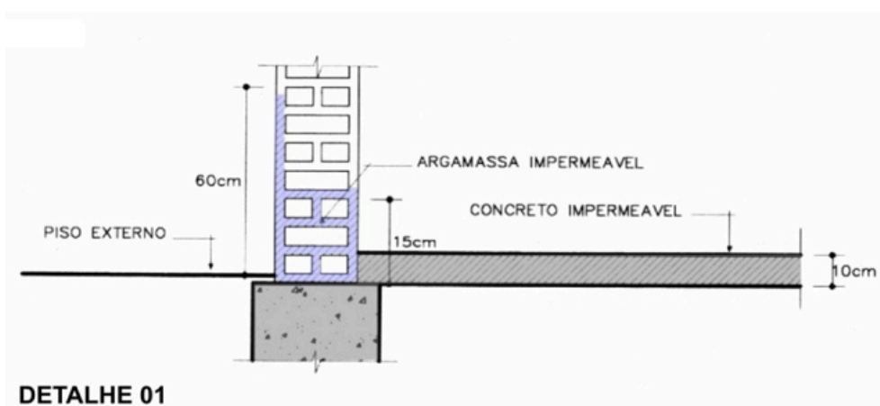
Figura 1: Detalhe 1 da impermeabilização do embasamento
