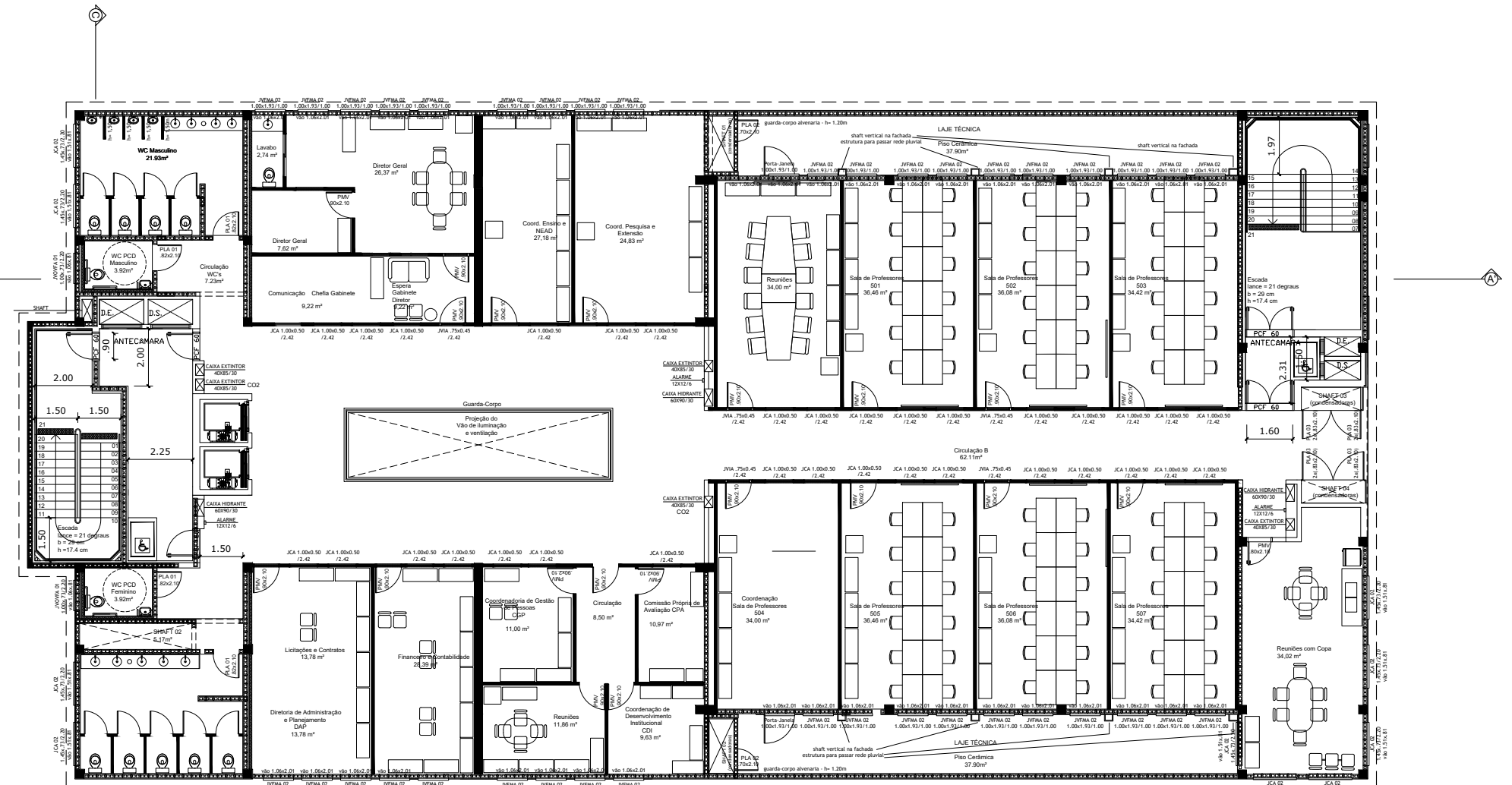
5º Pavimento A = 1063,35 m²
