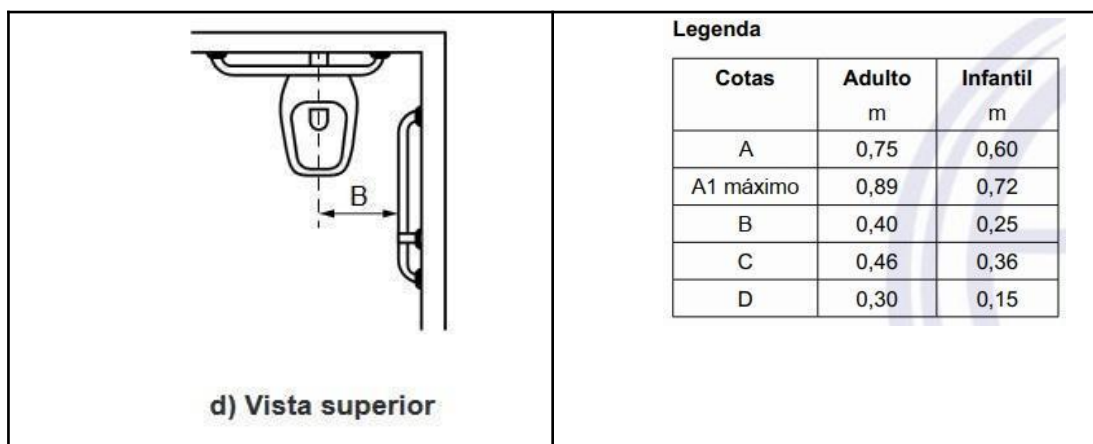
Figura 26: Detalhe da NBR 9050 - Bacia com caixa acoplada com barras de apoio ao fundo e a 90° na parede lateral
