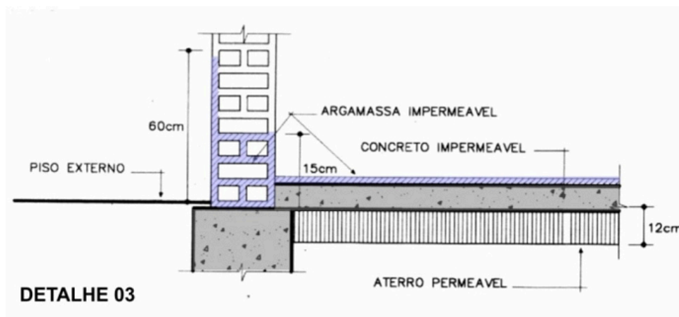
Figura 3: Detalhe 3 da impermeabilização do embasamento
