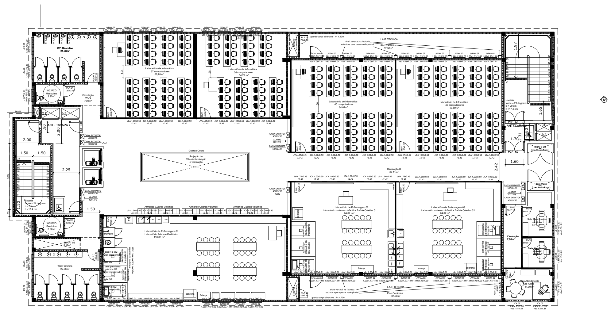
4º Pavimento A = 1063,35 m²
