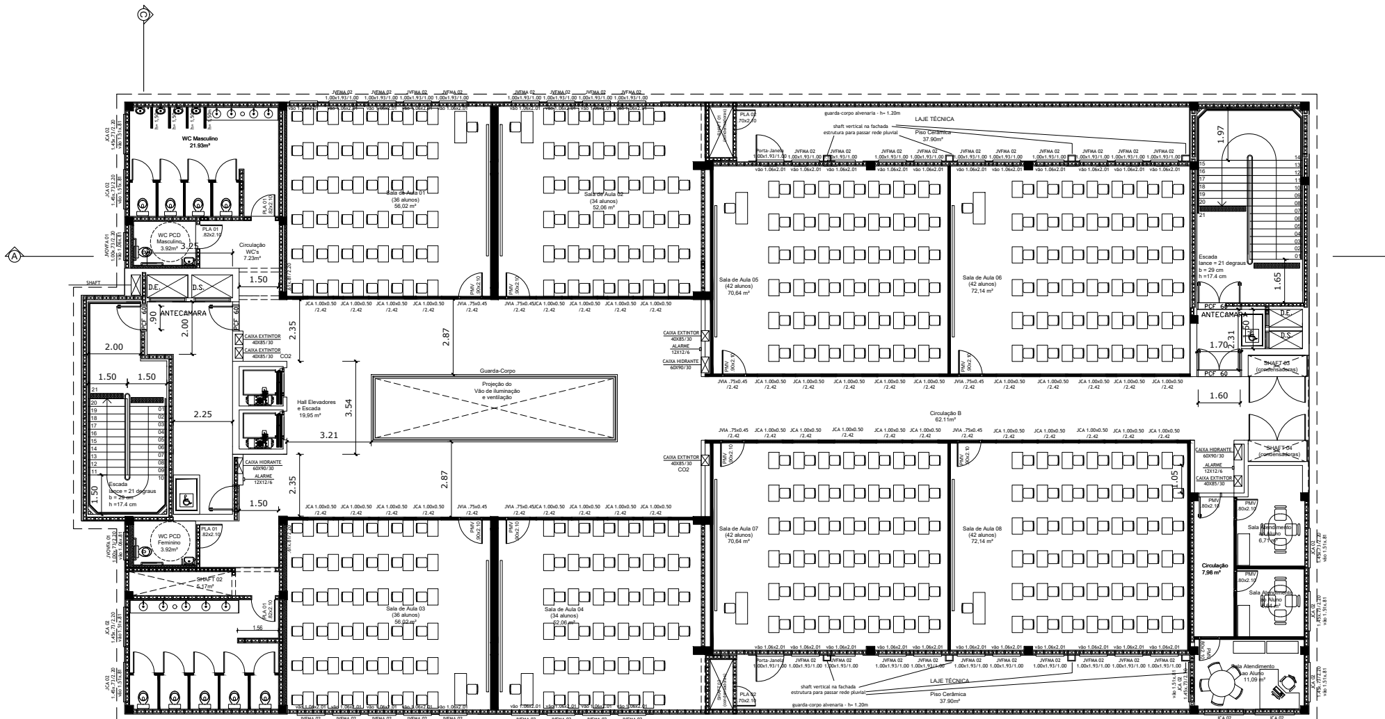
2º Pavimento A = 1063,35 m²
