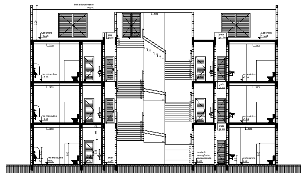
Corte CC'
