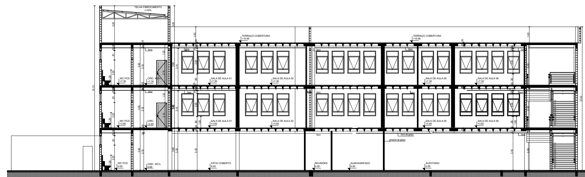
Corte AA'
