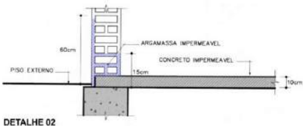
Figura 2: Detalhe 2 da impermeabilização do embasamento
