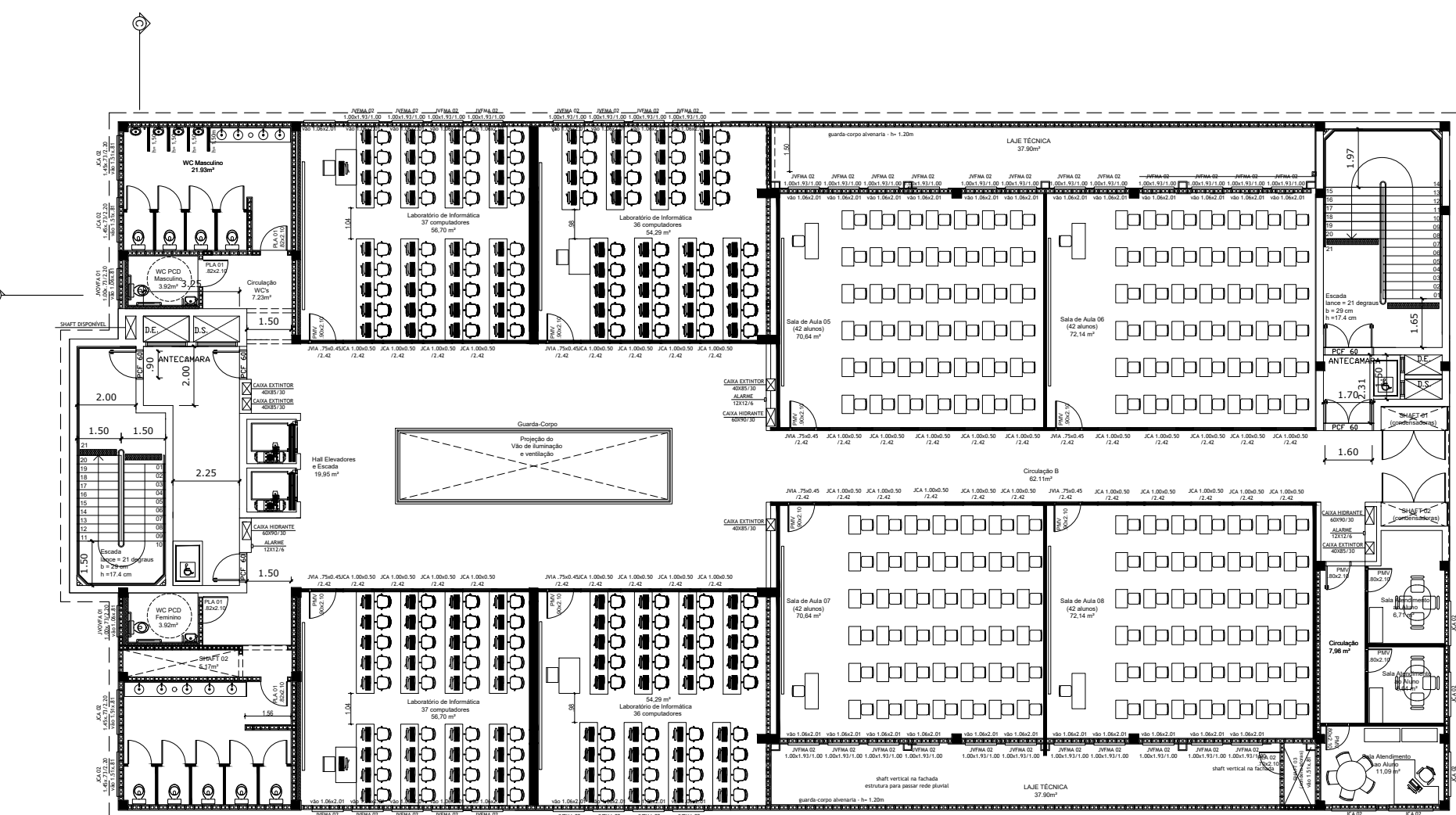
2º Pavimento A = 1063,35 m²
