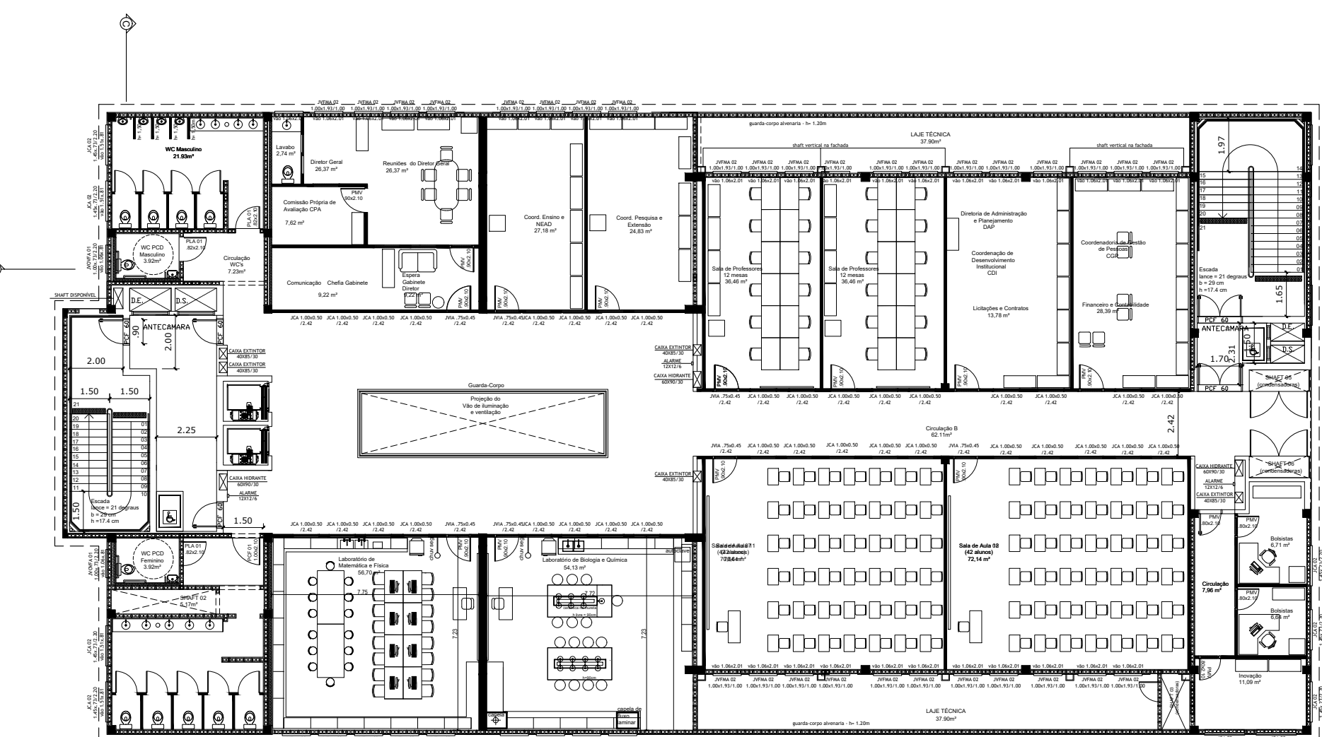
3º Pavimento A = 1063,35 m²
