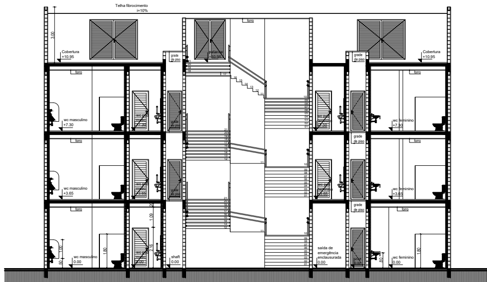
Corte CC'
