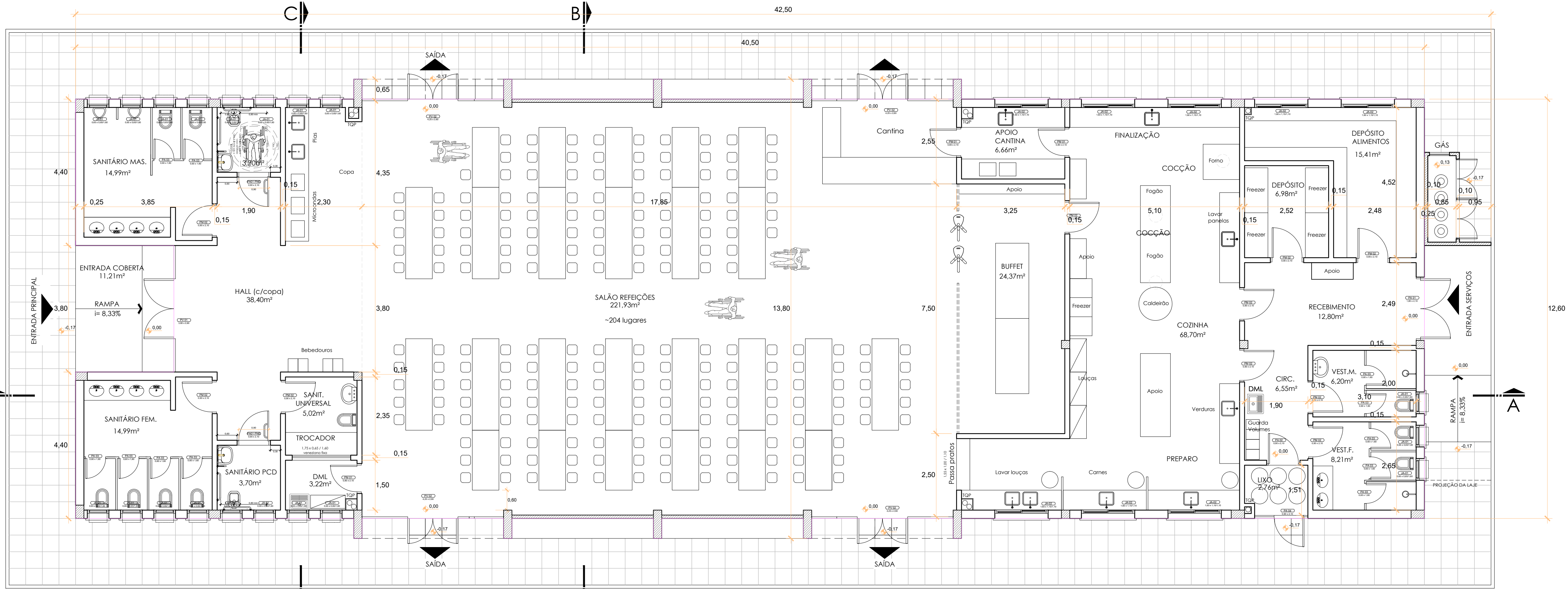
REFEITÓRIO PLANTA BAIXA ESCALA: 1/75 A= 500,59 m²
