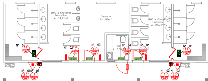
PLANTA BAIXA - LAYOUT ESC.: 1/50
